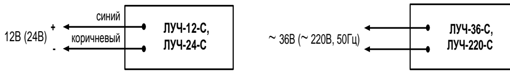
Рис.1. Схемы подключения.
